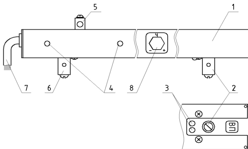
Рисунок 1.3 Конструкция ПРМ.
